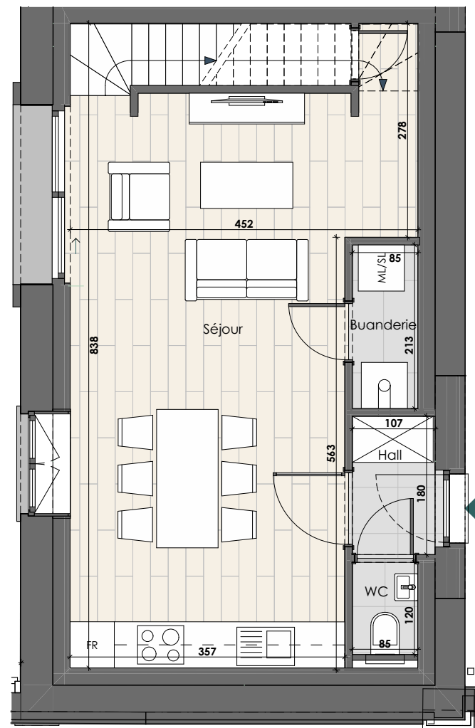
REZ-DE-JARDIN
